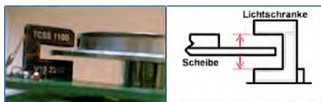
Abbildung 14 Ausrichtung der Sektorscheibe in der Lichtschranke
